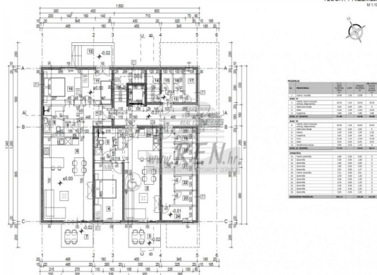
TLOCRT PRIZEMLIJA M 1:100
